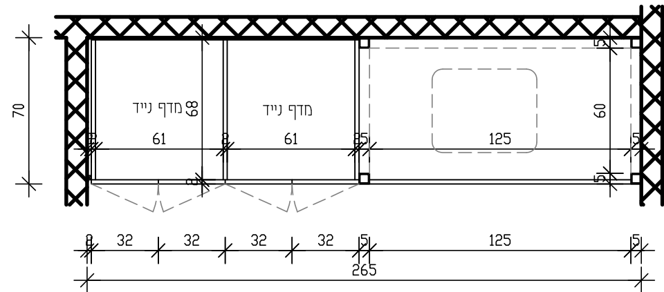
תוכנית מתחת המשטח קנ"מ 1:25
