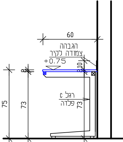
חתך א-א קנ"מ 25:
