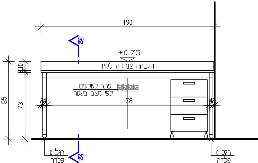
חזית המשטח קנ"מ 25:
