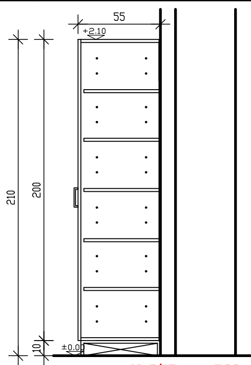
חתך א-א קנ"מ 1:25
