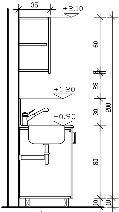
חתך א-א קנ"מ 25
