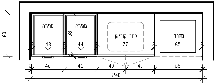
תוכנית מתחת המשטח קנ"מ 25
