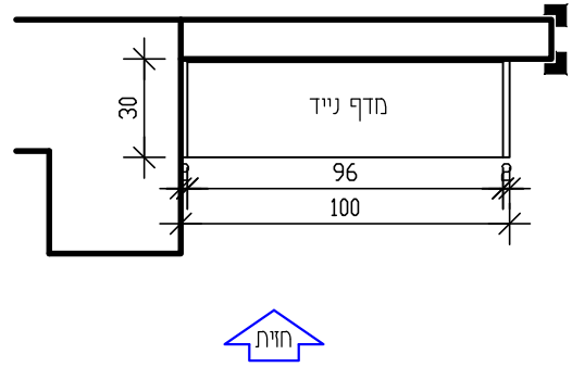
תוכנית מגירות קנ"מ 1:25
