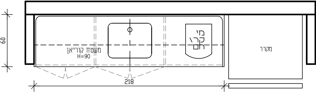
תוכנית מעל המשטח קנ"מ 1:25
