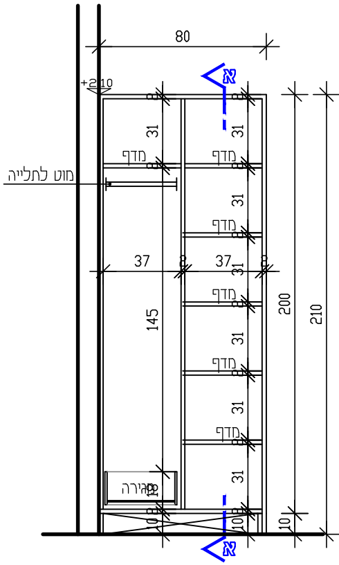
חזית פנימית קנ"מ 25
