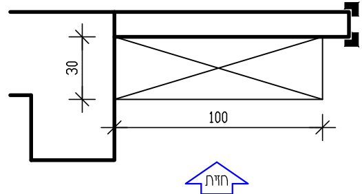
תוכנית מעל המשטח קנ"מ 1:25
