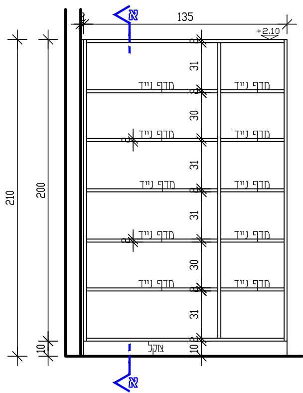
חזית פנימית קנ"מ 1:25
