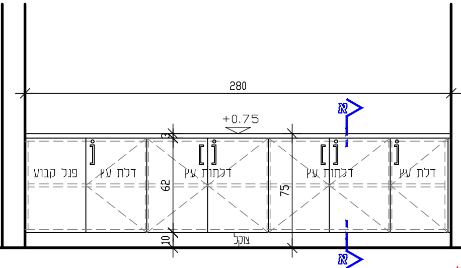
תוכנית מתחת המשטח קנ"מ 1:25
