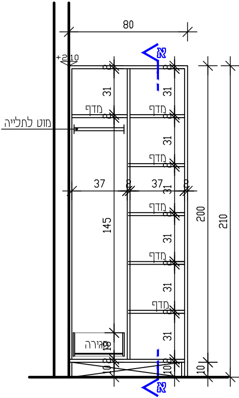
חזית פנימית קני' 25'
