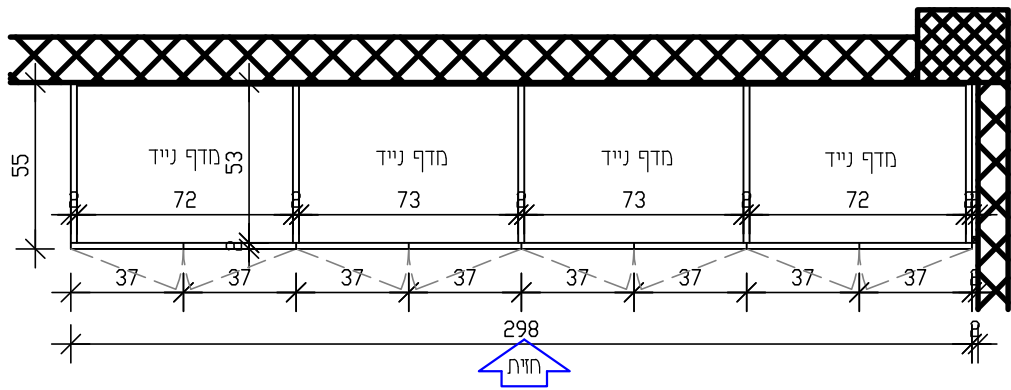
תוכנית מתחת המשטח קנ"מ 1:25
