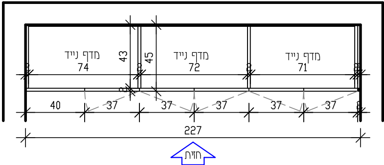
תוכנית מתחת המשטח קנ"מ 1:25
