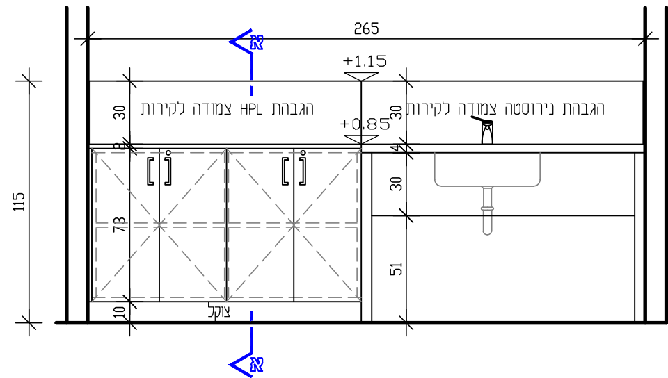
חזית המשטח קנ"מ 1:25
