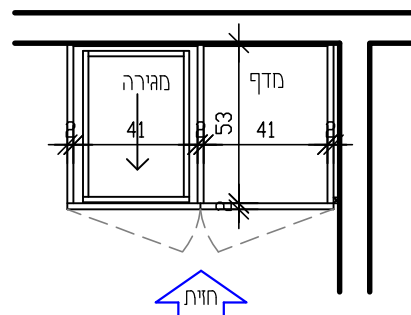
תוכנית מתחת המשטח קנ"מ 25:
