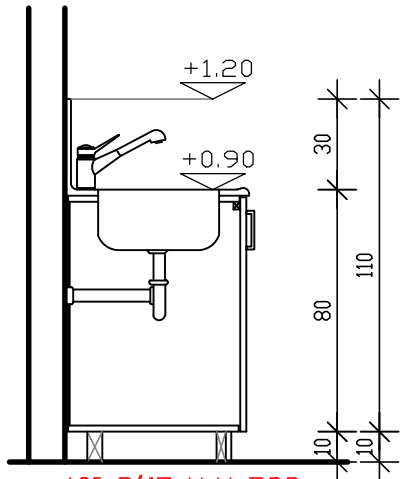
חתך א-א קנ"מ 25:1
