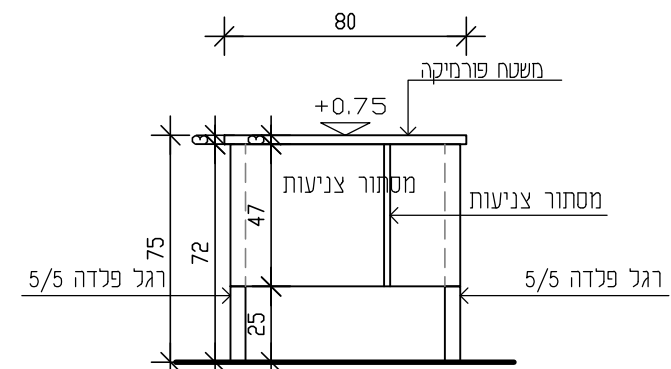
חתך א-א שולחן קנ"מ 25:
