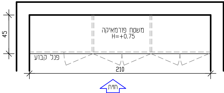
תוכנית מעל המשטח קנ"מ 1:25
