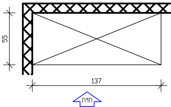
תוכנית מעל המשטח קנ"מ 1:25
