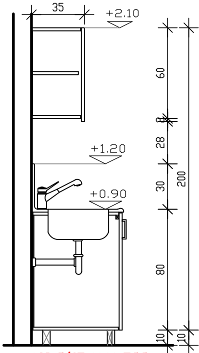
חתך א-א קנ"מ 1:25
