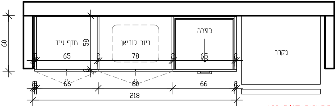
תוכנית מתחת המשטח קנ"מ 1:25
