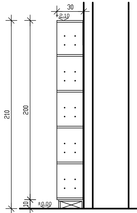
חתך א-א קנ"מ 1:25
