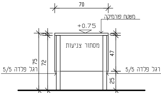
חַתָּךְ א-א שולחן קנ"מ 25
