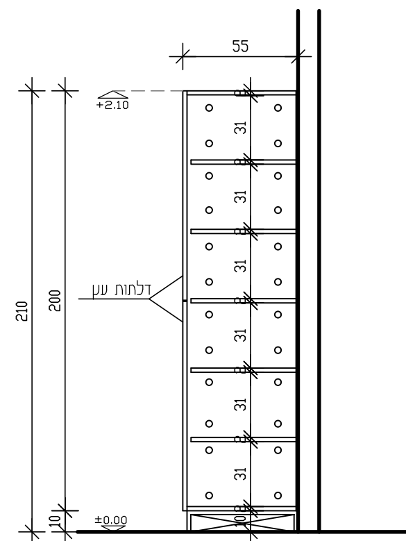
חתך א-א קנ"ח 25:
