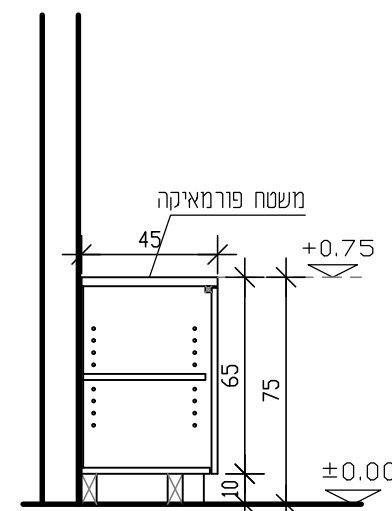
חתך א-א ארון קנ'ם 25:
