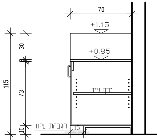
חתך א-א קנ"מ 1:25
