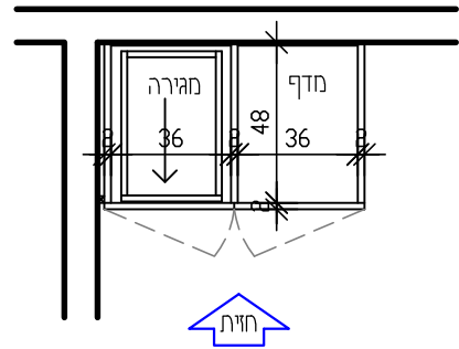
חזית פנימית קנ"מ 25
