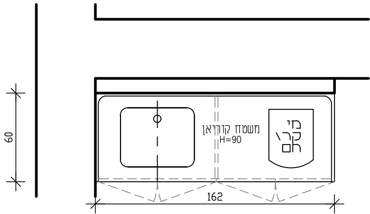
תוכנית מעל המשטח קנ"מ 25:1
