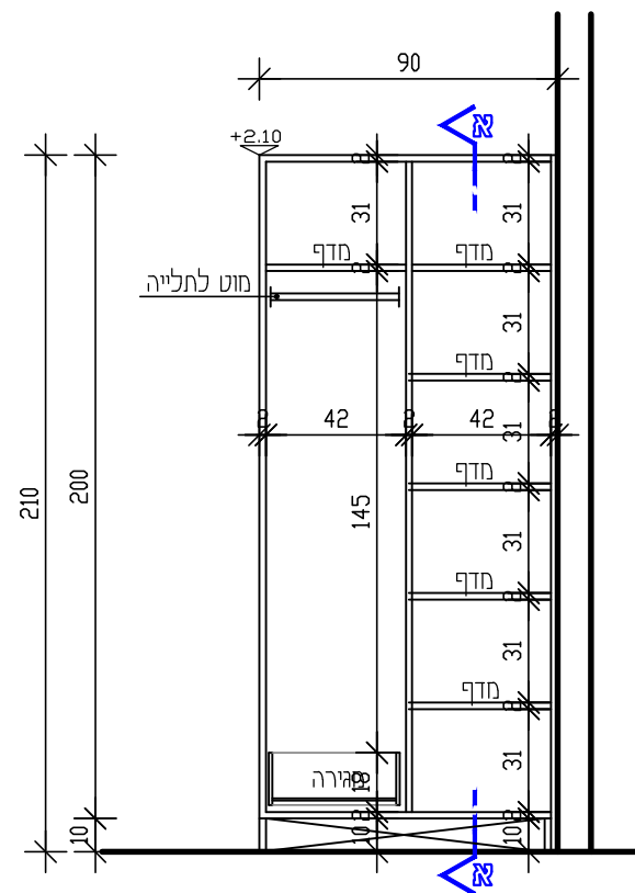
חזית פנימית קנ"מ 25:
