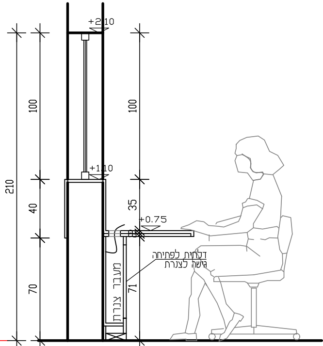
חתך א-א קנ"מ 1:25
