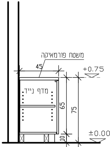
חתך א-א קנ"מ 1:25
