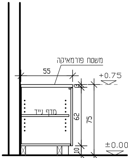
חתך א-א קנ"מ 1:25
