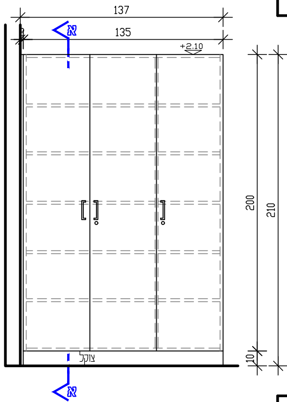
חזית חיצונית קנ"מ 1:25
