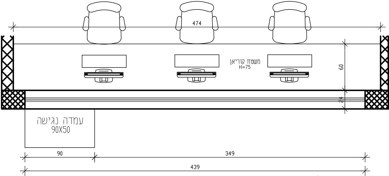
תוכנית מעל המשטח קנ"מ 1:25
