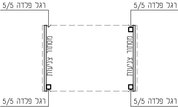
תוכנית מעל המשטח קנ"מ 25
