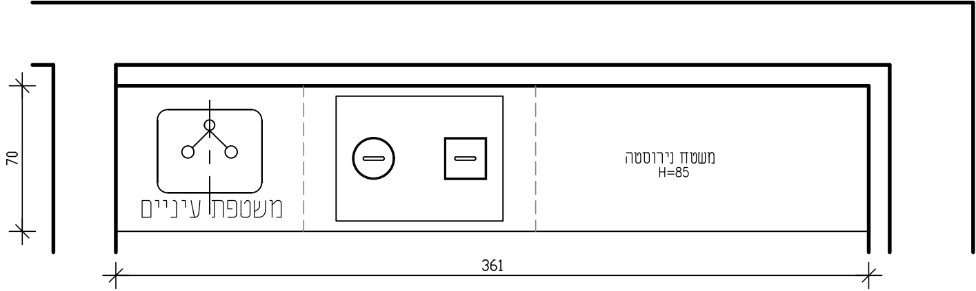
תוכנית מעל המשטח קנ"מ 1:25
