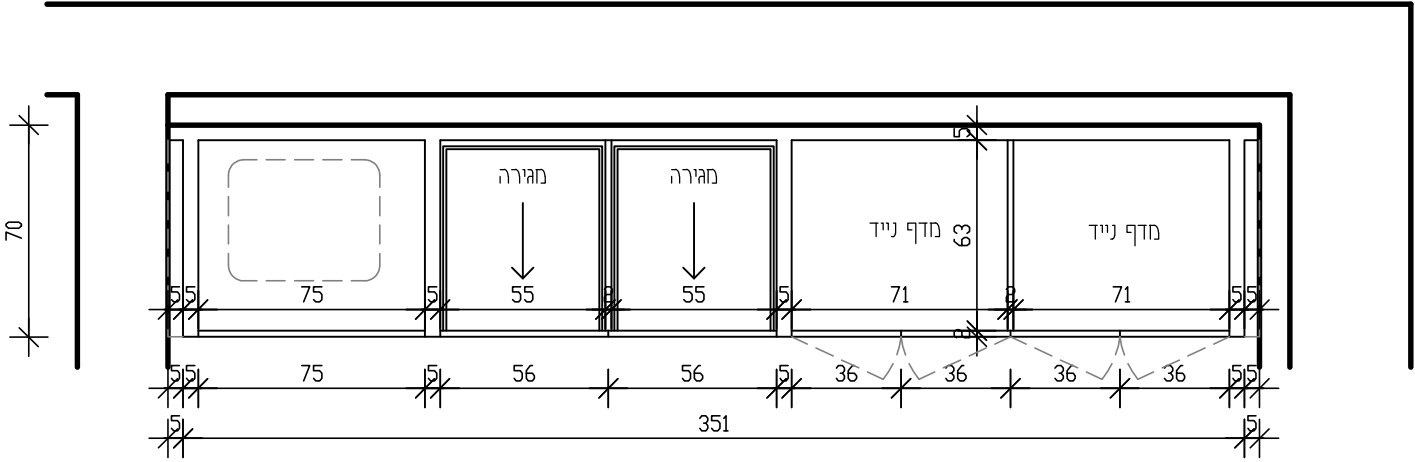
תוכנית מתחת המשטח קנ"מ 1:25
