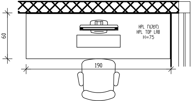
תוכנית מעל המשטח קנ"מ 25:
