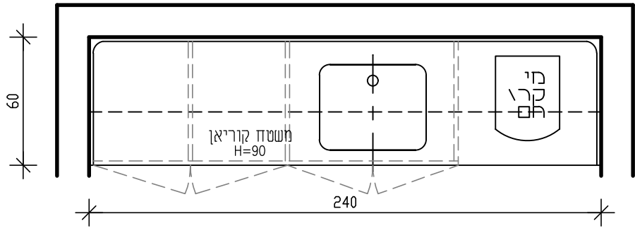
תוכנית מעל המשטח קנ"מ 25
