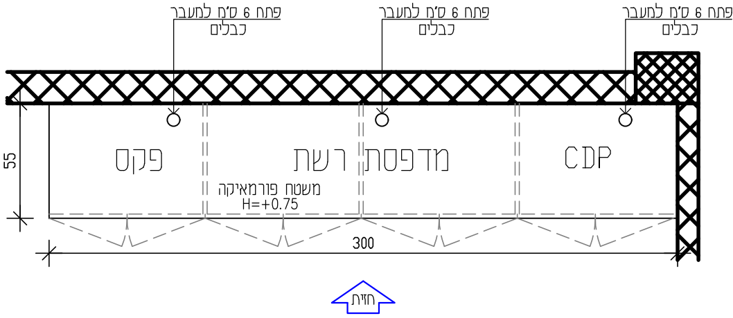
תוכנית מעל המשטח קנ"מ 1:25
