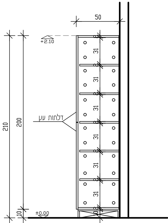
חזית חתך א-א קנ"מ 25
