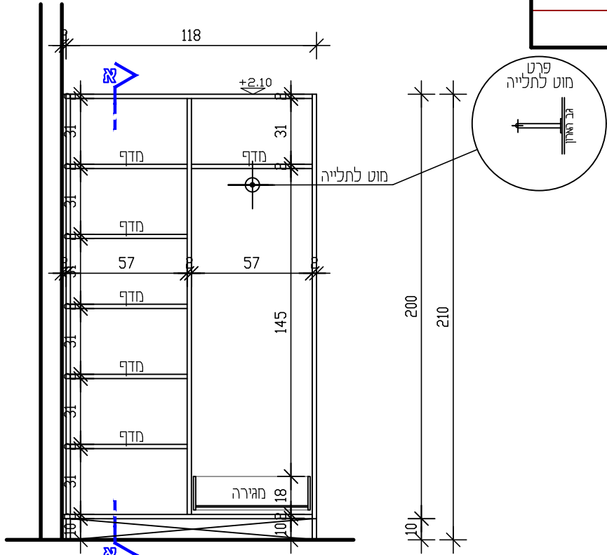
חזית פנימית קנ"מ 25
